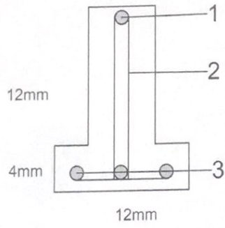
CHAPEAU DES NERVURES T_{12} = \text{Min } L/4
