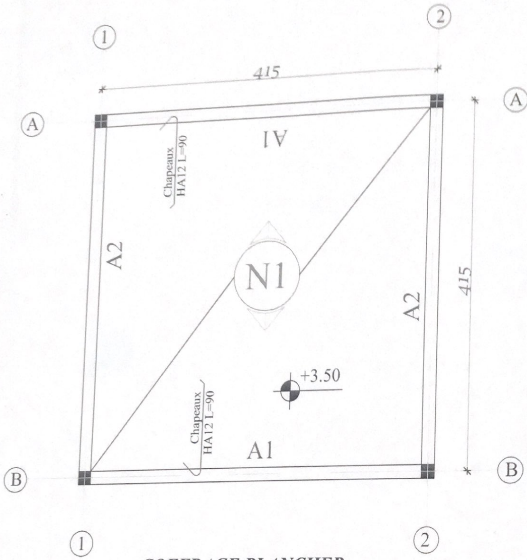
COFFRAGE PLANCHER
