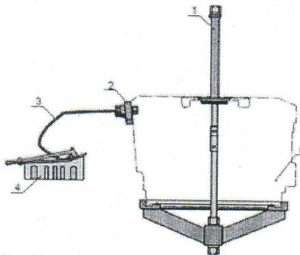
Fig 12-14 Dispositif d'essai de pression
