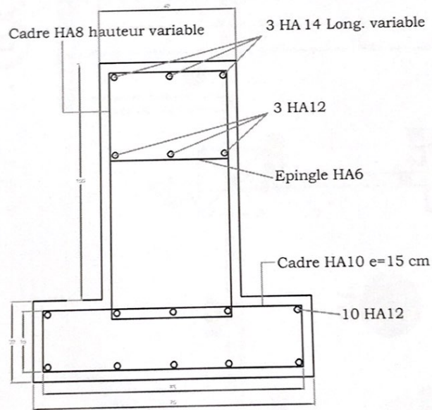
longrine sous rail
