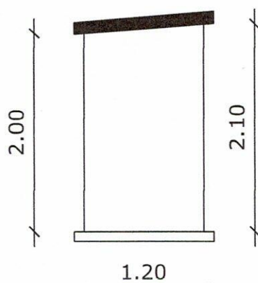
façade latérale
