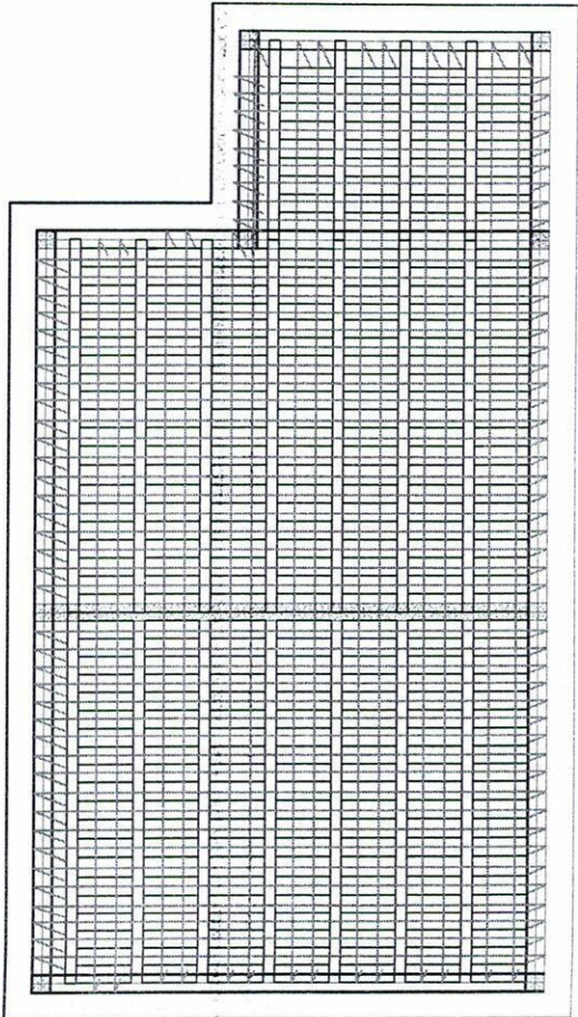
DALLE SUPÉRIEURE EN HOURDIS CREUX 0.60/0.20 AVEC POSE TREILLIS EN FER Ø8 écartement 15/15 l'ensemble est accroché sur des éléments préfabriqués en BA avec fer Ø12
