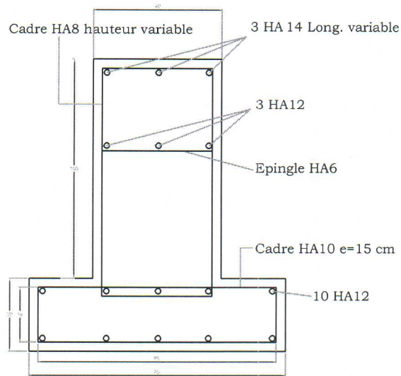
longrine sous rail
