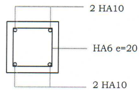
Chaînage Bas et Haut (20x20)
