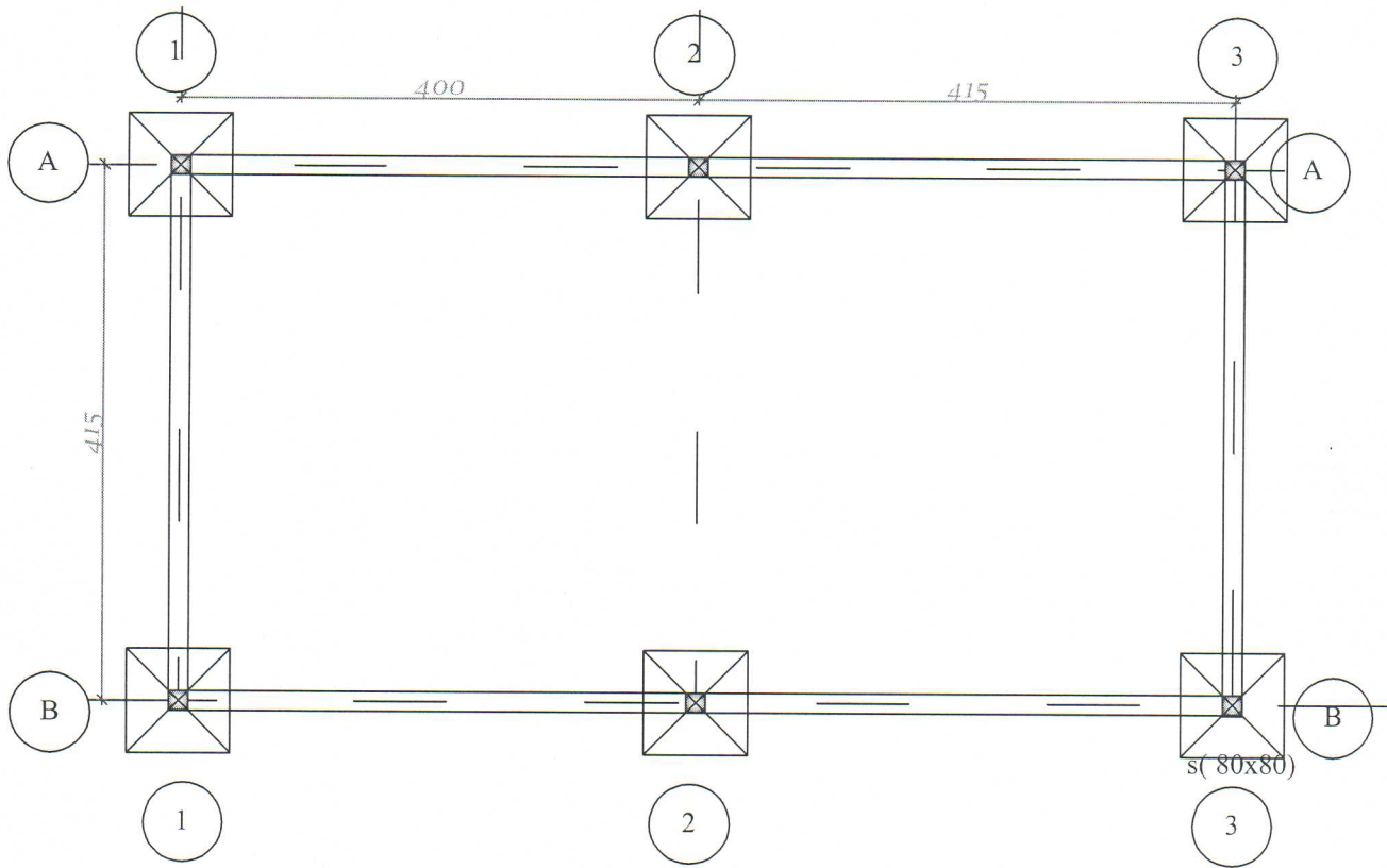
PLAN FONDATION
